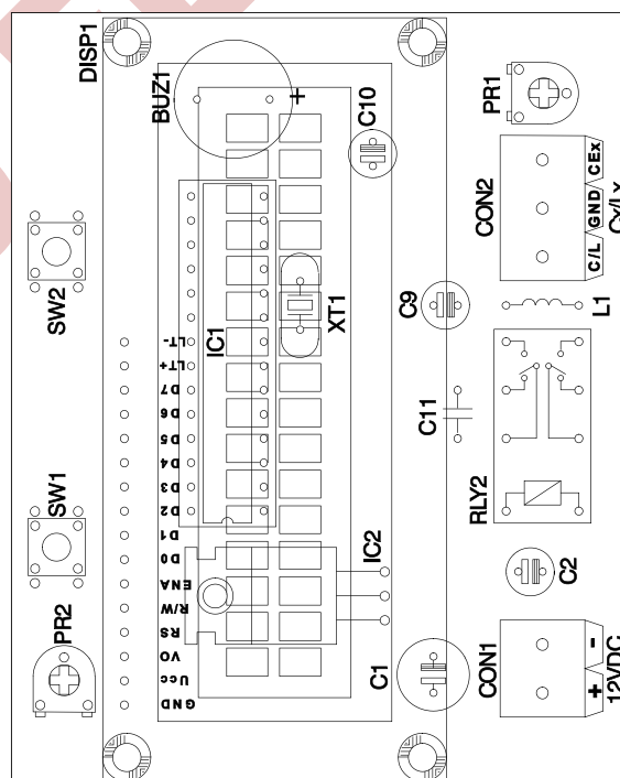
Rysunek 2. Schemat montażowy płytki bazowej (elementy przewlekane)
