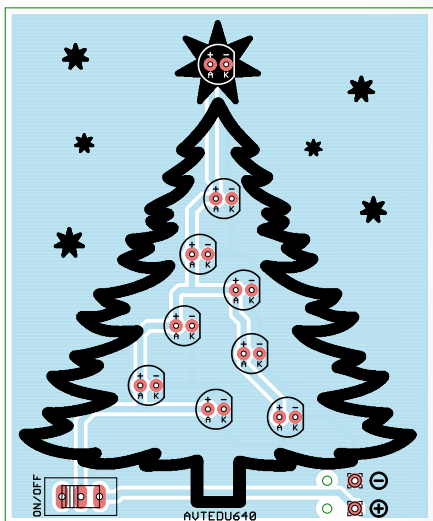
Rys. 2 Rozmieszczenie elementów na płytce drukowanej
