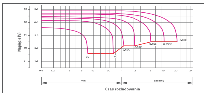
CHARAKTERYSTYKA ROZŁADOWANIA
