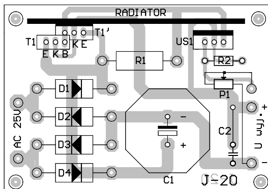
Schemat montażowy
